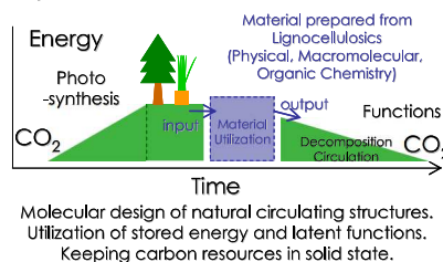
図. エネルギー、時間、機能の軸から考える炭素循環の概念図
